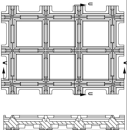
SECTION V-V SCALE 2:1
