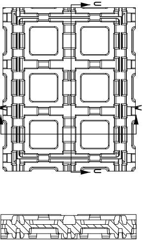
SECTION V-V SCALE 2:1
